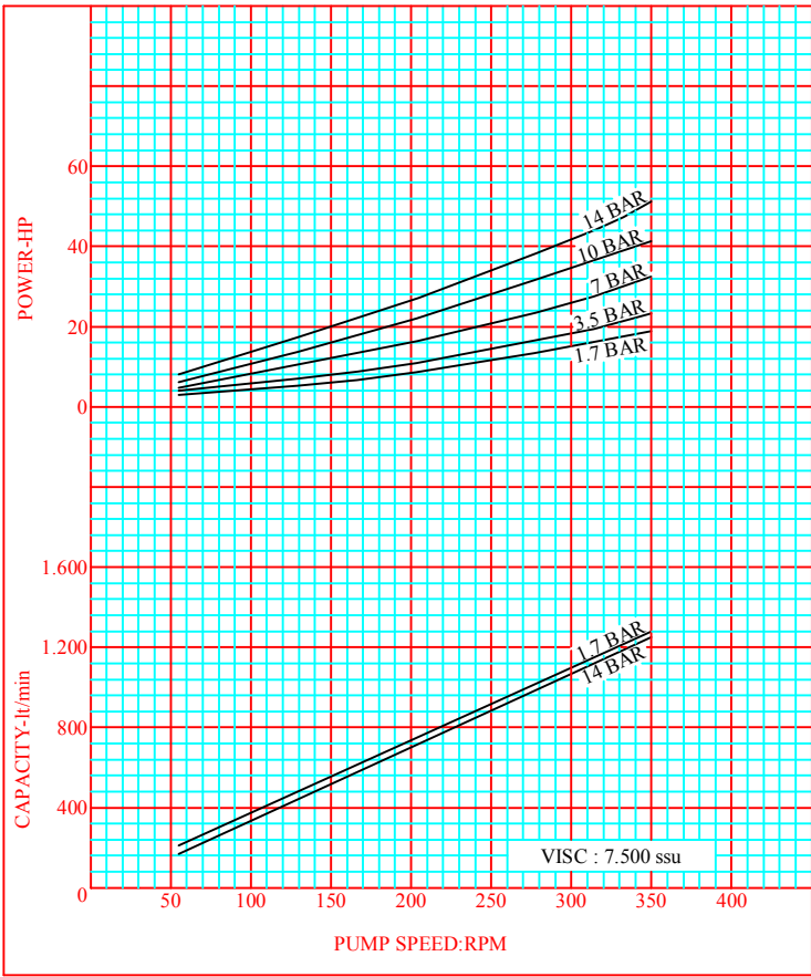
CURVE NO:AK-05
