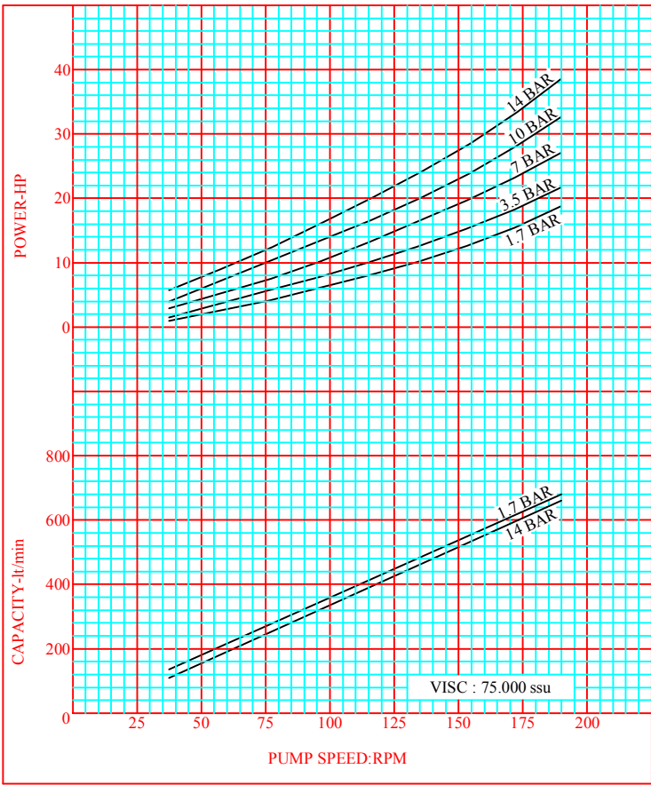
CURVE NO:AK-07
