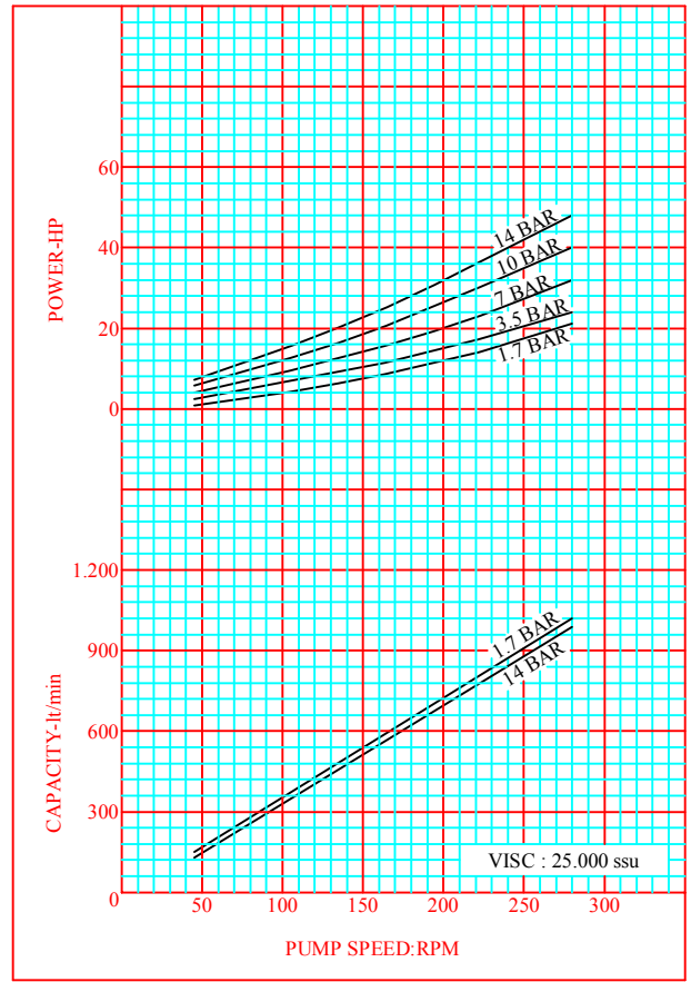
CURVE NO:AK-06
