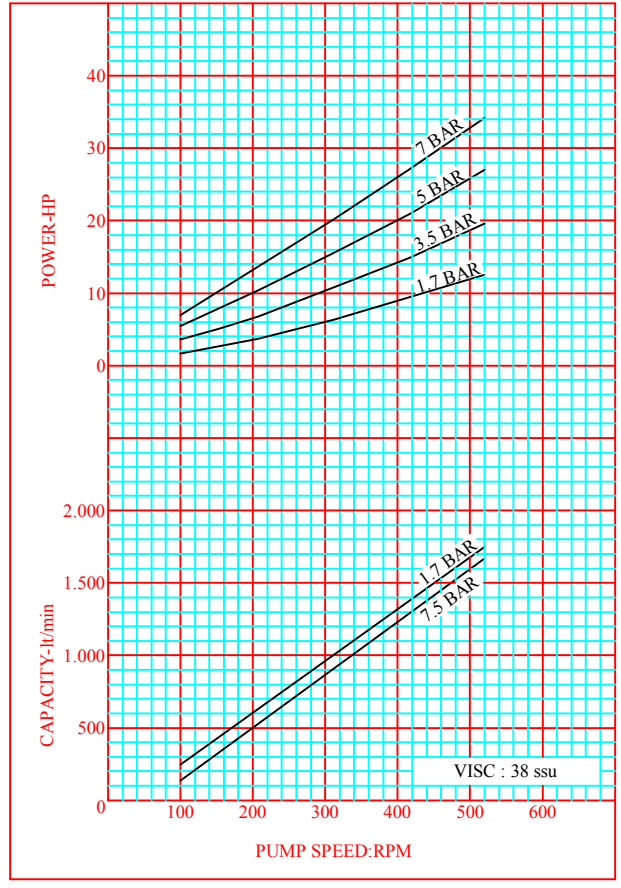
CURVE NO:AK-01
