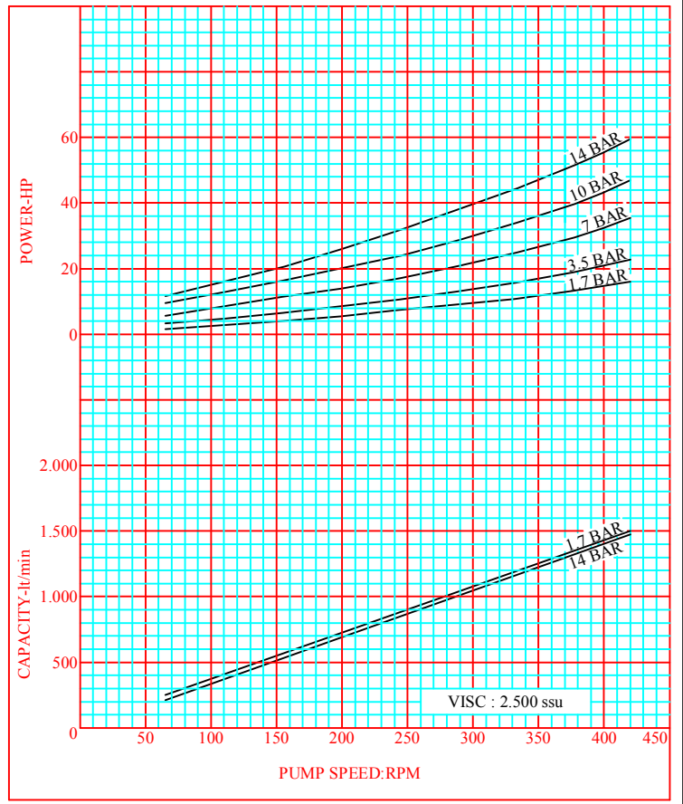
CURVE NO:AK-04
