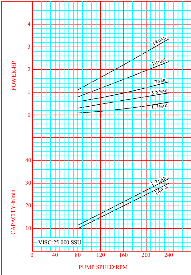
CURVE NO:CDK-07
