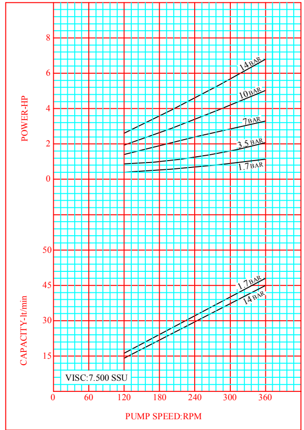
CURVE NO:CDK-06
