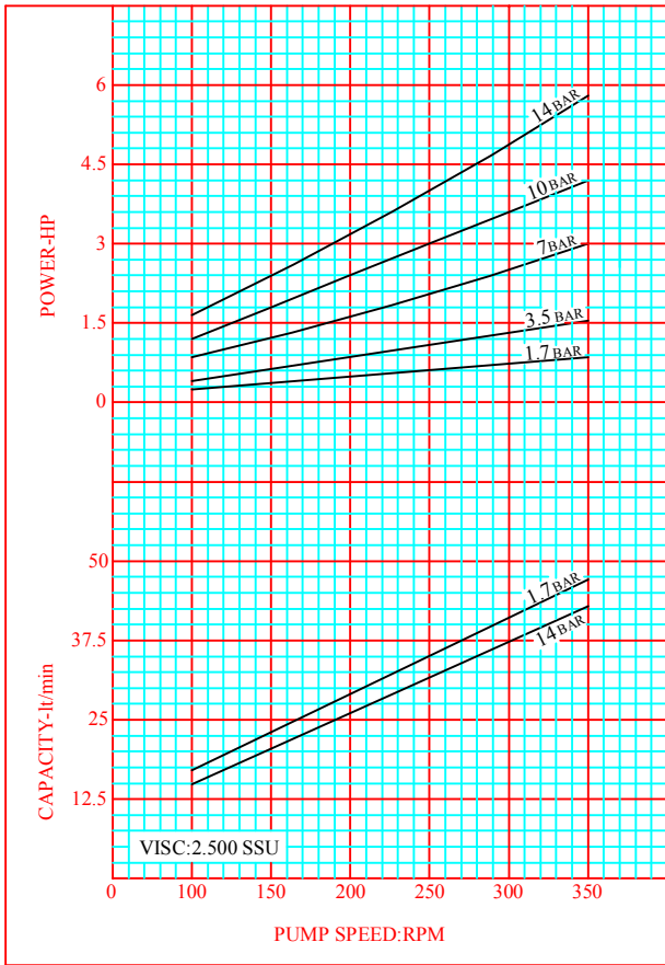
CURVE NO:CDK-05
