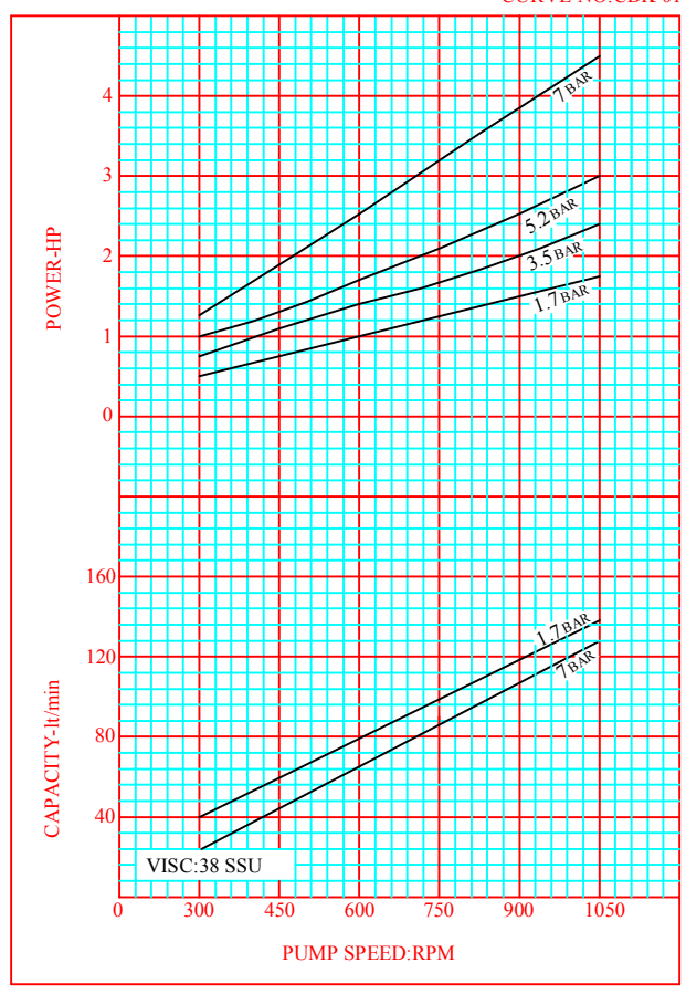
CURVE NO:CDK-01
