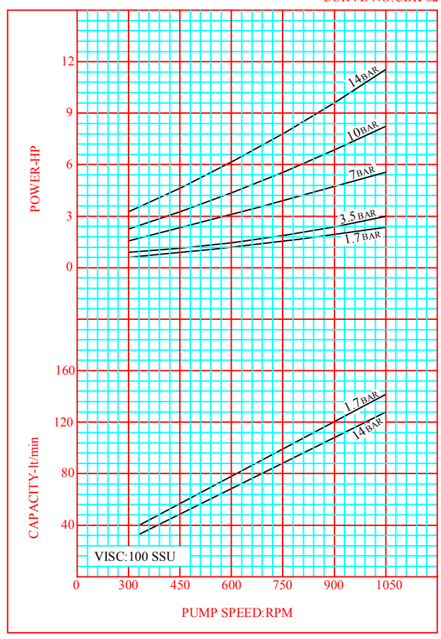
CURVE NO:CDK-02
