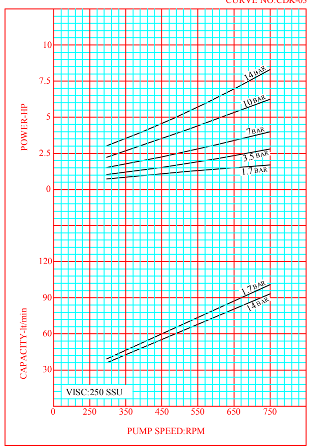
CURVE NO:CDK-03
