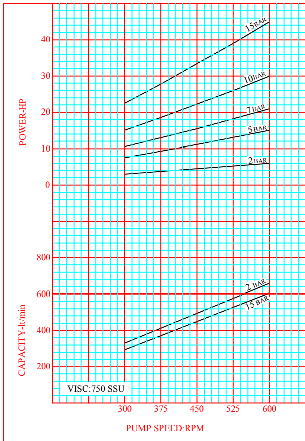
CURVE NO:XLA-03
