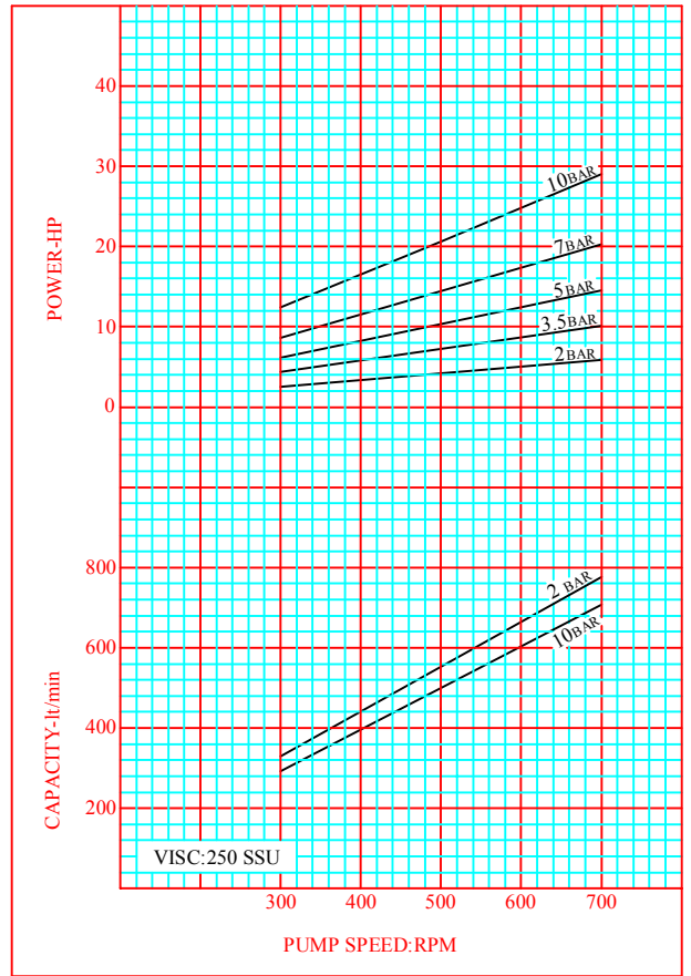
CURVE NO:XLA-02
