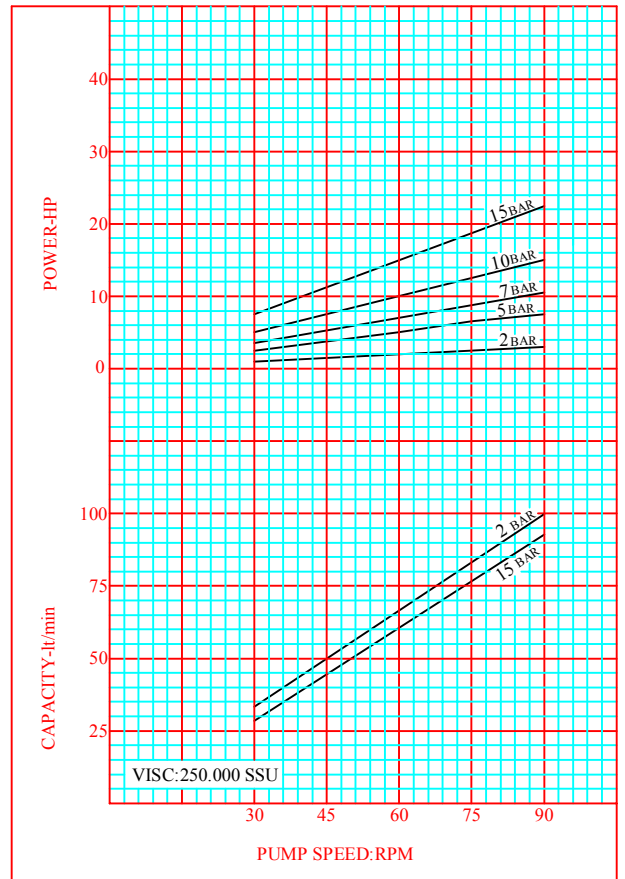
CURVE NO:XLA-08
