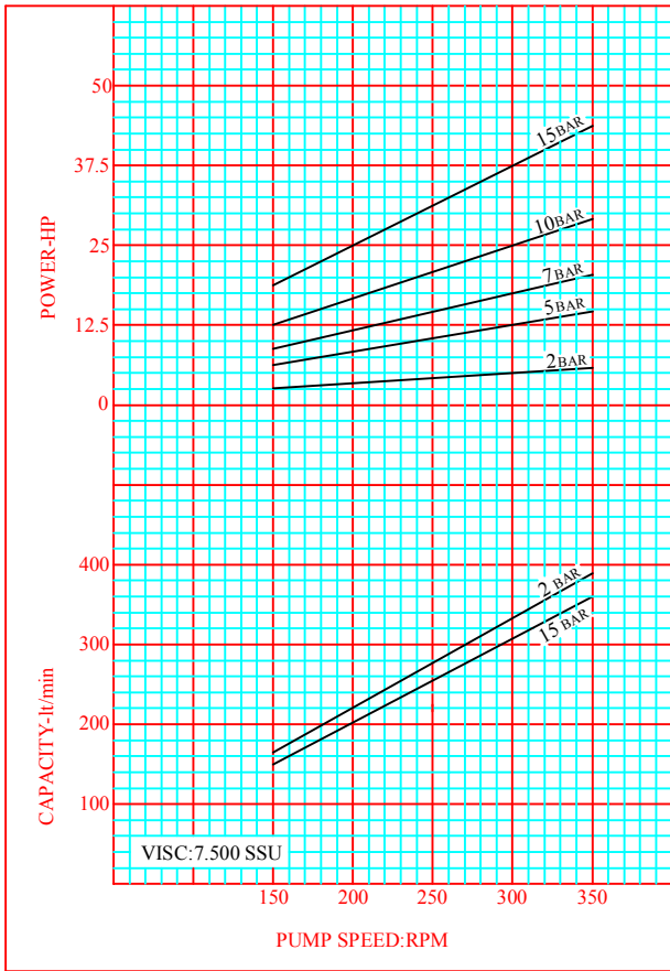
CURVE NO:XLA-05
