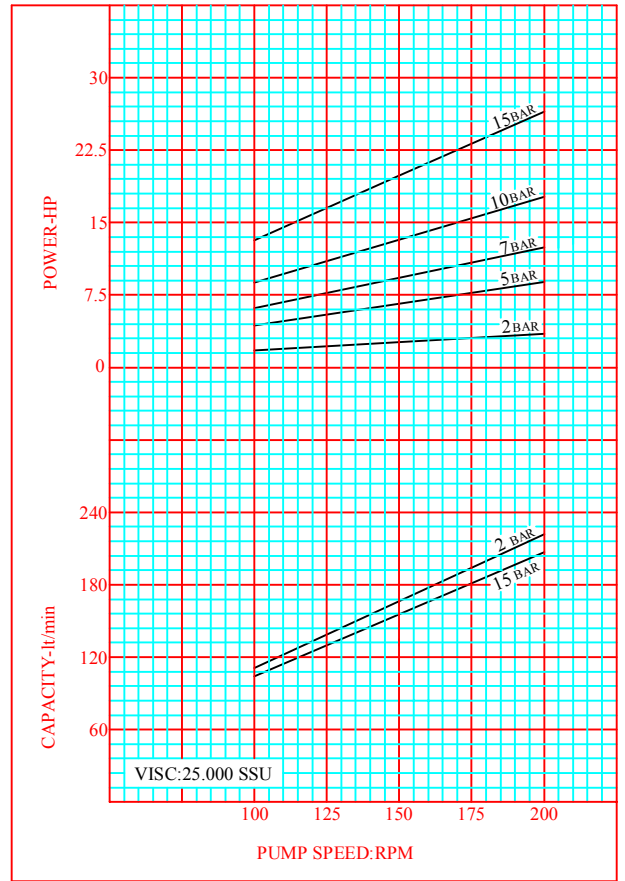
CURVE NO:XLA-06
