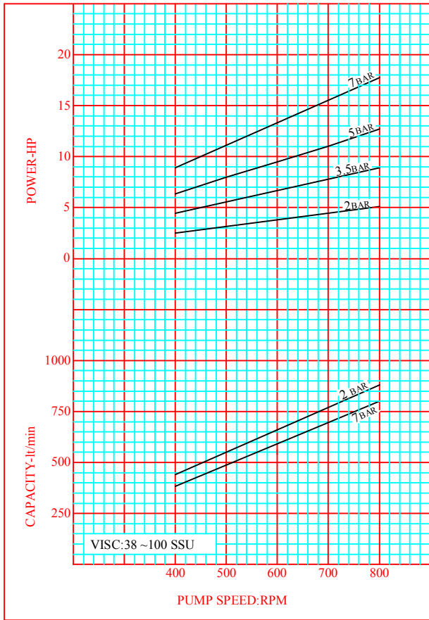
CURVE NO:XLA-01
