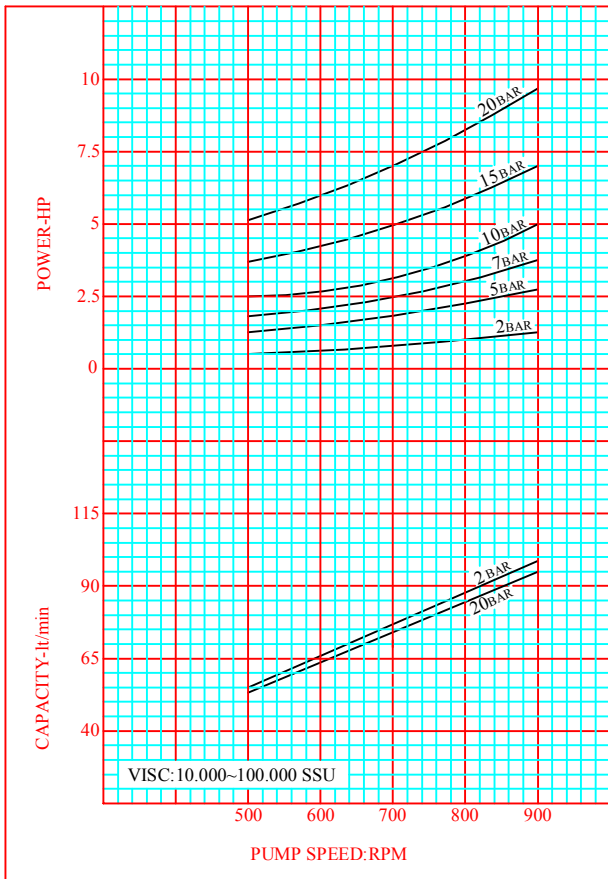
CURVE NO:XLAK-03
