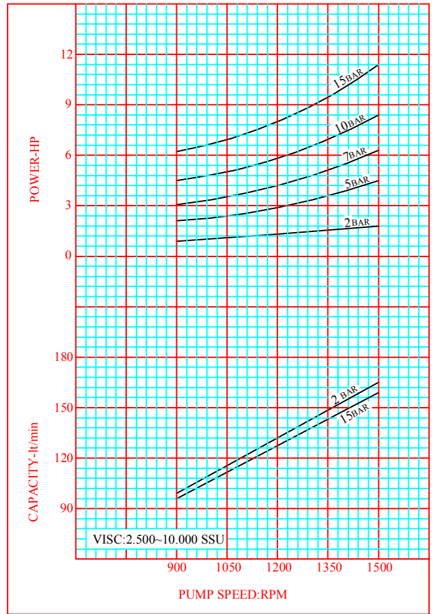
CURVE NO:XLAK-02
