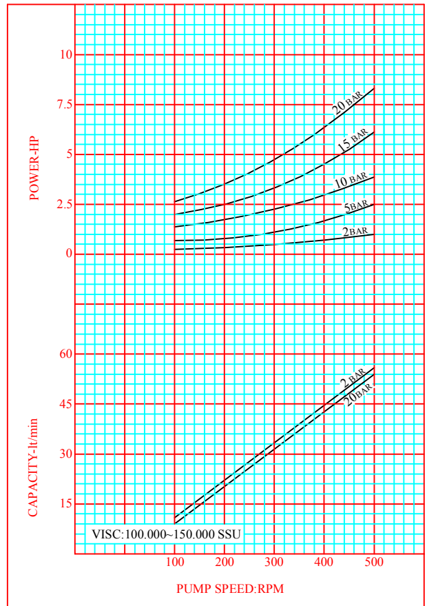
CURVE NO:XLAK-04
