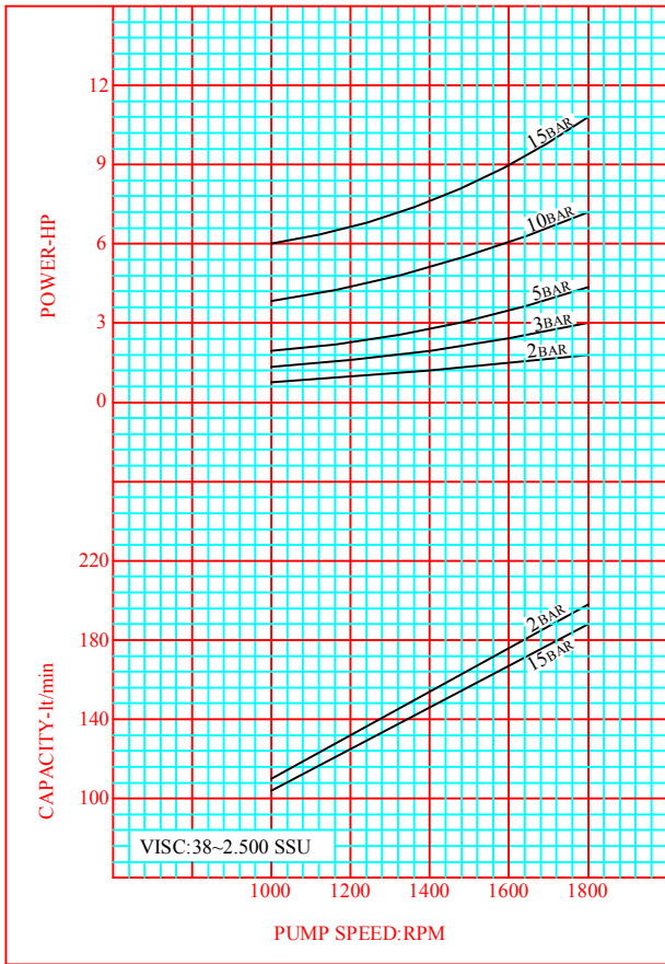
CURVE NO:XLAK-01
